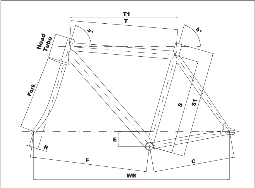
Battuta mozzo posteriore 120mm - Rear hub dimension 120mm
